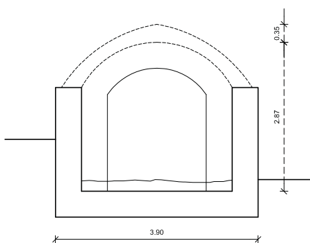
SECCION
