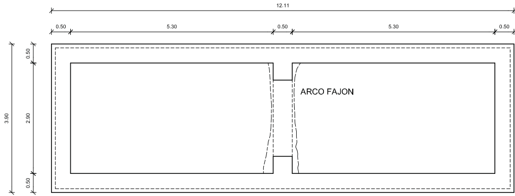
PLANTA VASO
