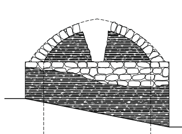
FACHADA NORTE
