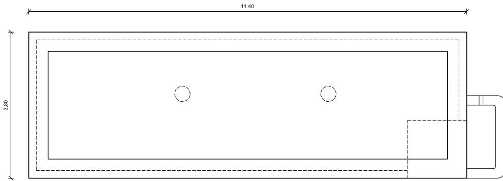
PLANTA VASO
