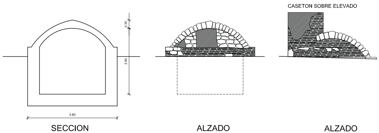
ALZADOS
