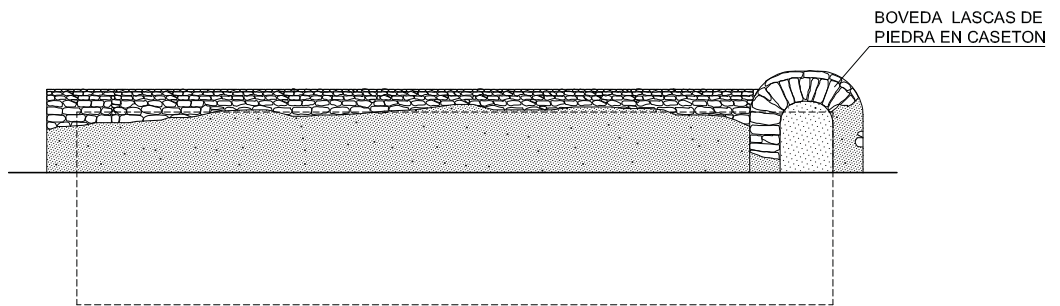
ALZADO LATERAL
